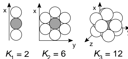
Piešinys 2. Kissing number iliustracija prie N = 1, 2, 3 .
